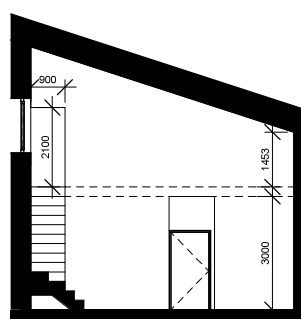
ANTRESOLĒS PJŪVIS
