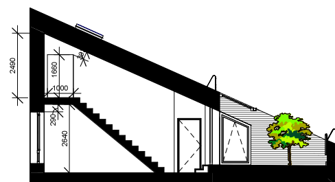
Antresolės pjūvis
