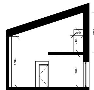
ANTRESOLĖS PJŪVIAI
