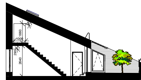
Antresolės pjūvis
