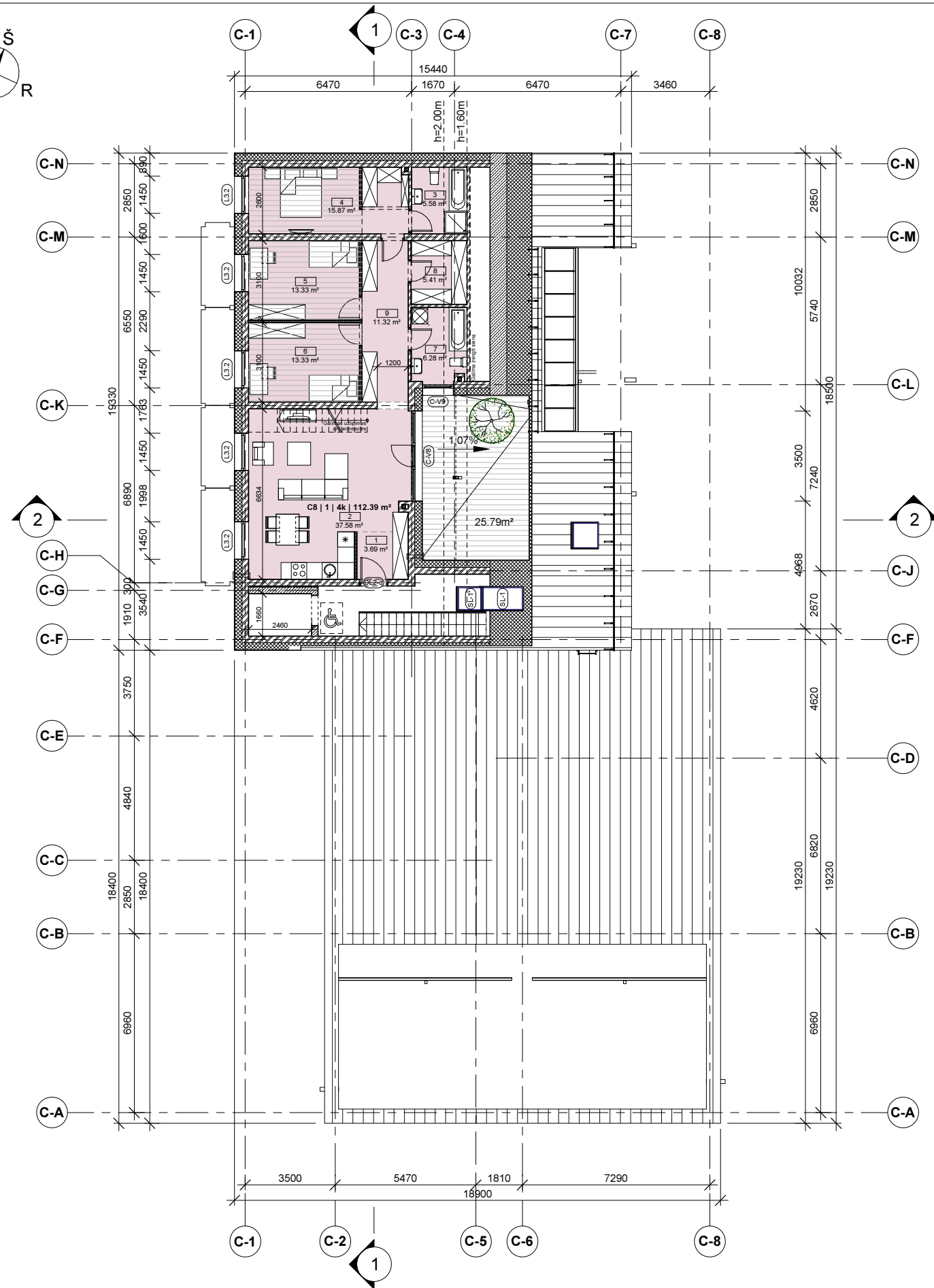
Antresolės planas
