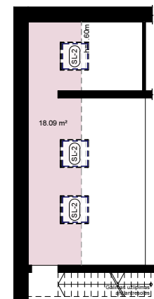
Antresolės planas
