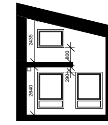
Antresolės pjūvis
