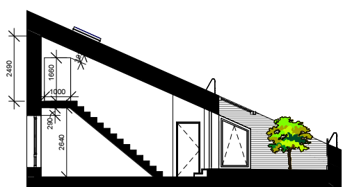
Antresolės pjūvis
