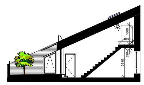
Antrosolės pjūvis
