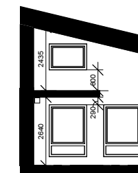
Antresolės pjūvis
