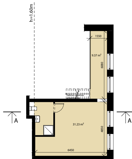
Antresolės planas
