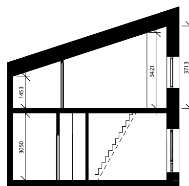
Antresolės pjūvis A-A
